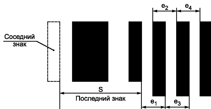
Рисунок 8 — Размеры вспомогательных шаблонов
